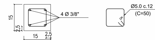
DETALHE FERRAGENS (15x15)
