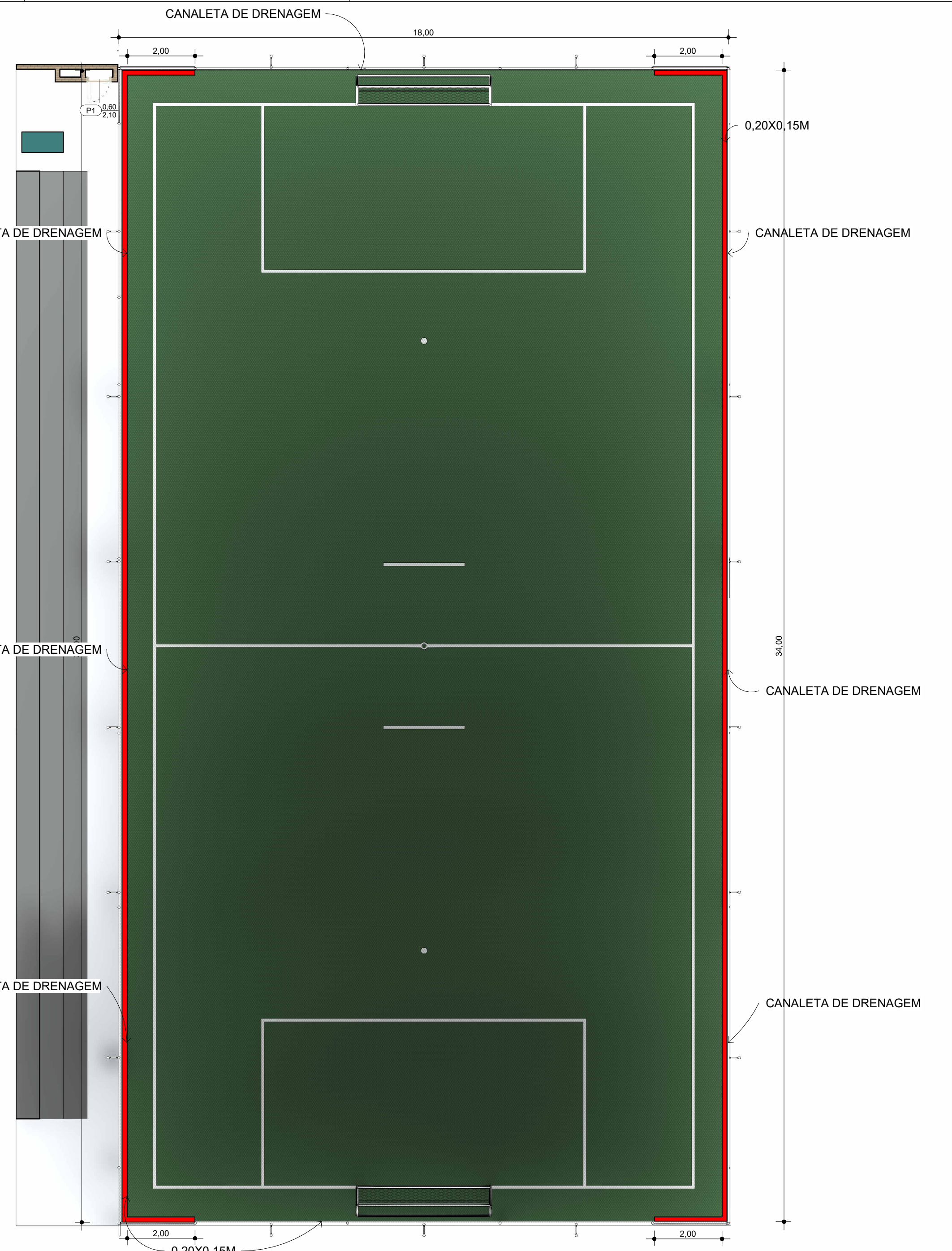
2 PLANTA BAIXA DRENAGEM 1 : 100
