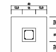
BLOCOS E PILARES
