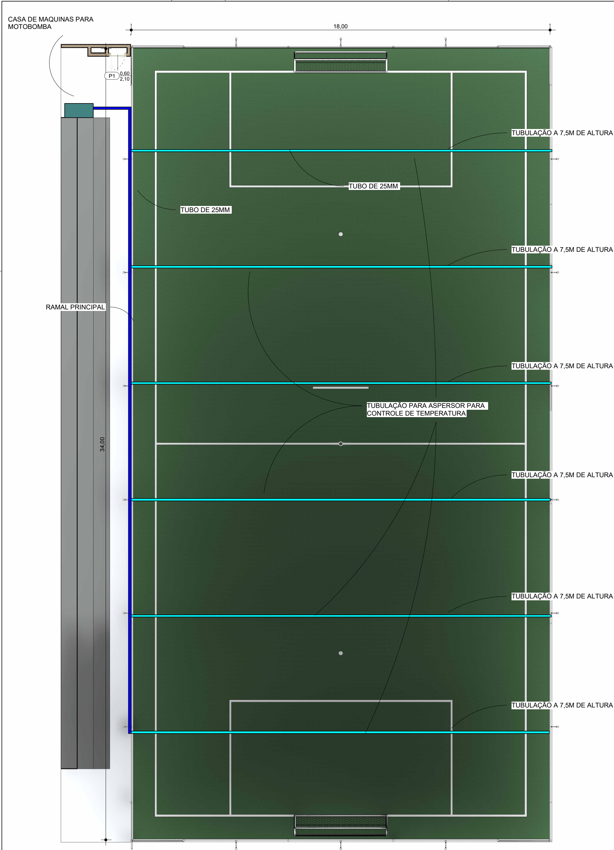
1 PLANTA BAIXA HIDRAULICA 1 : 100
