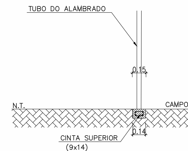
DETALHE DA CINTA PARA TRAVAMENTO DOS PILARES
