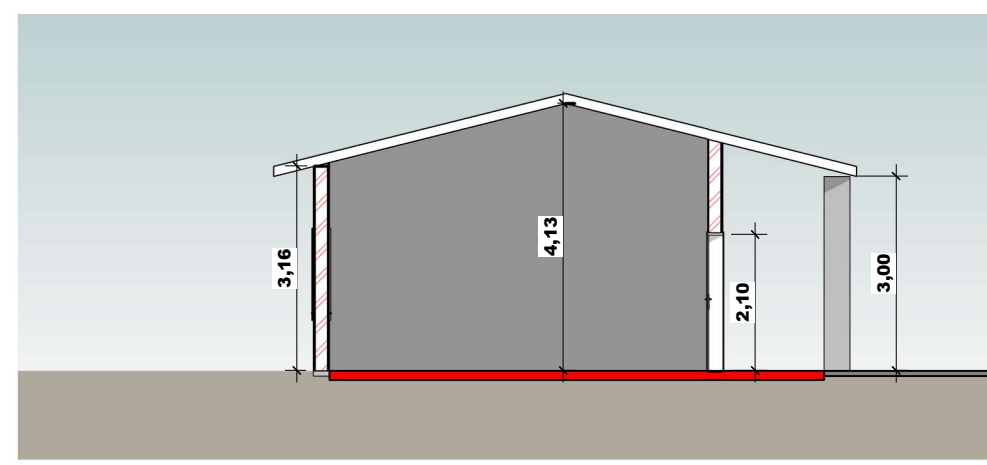
3 CORTE 02 1:75
