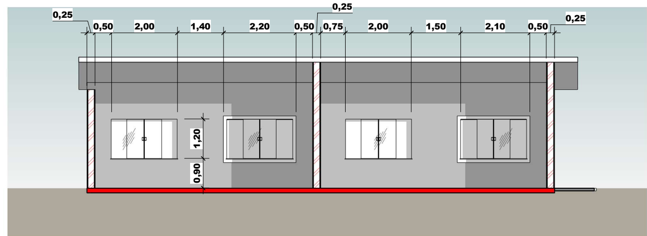
2 CORTE 01 1:75
