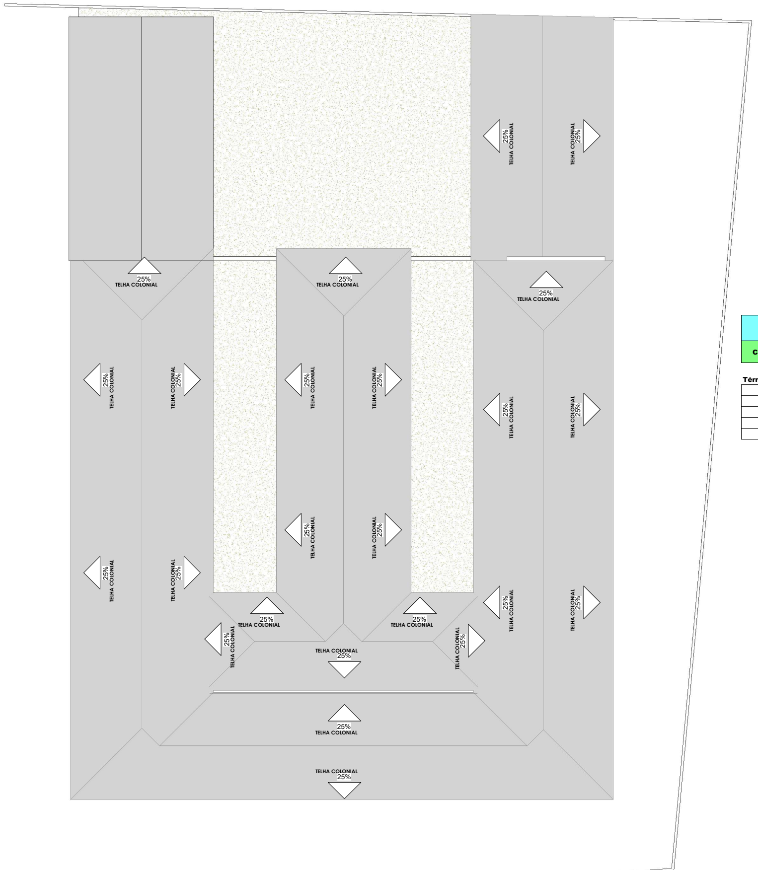
2 Cobertura 1 : 150
