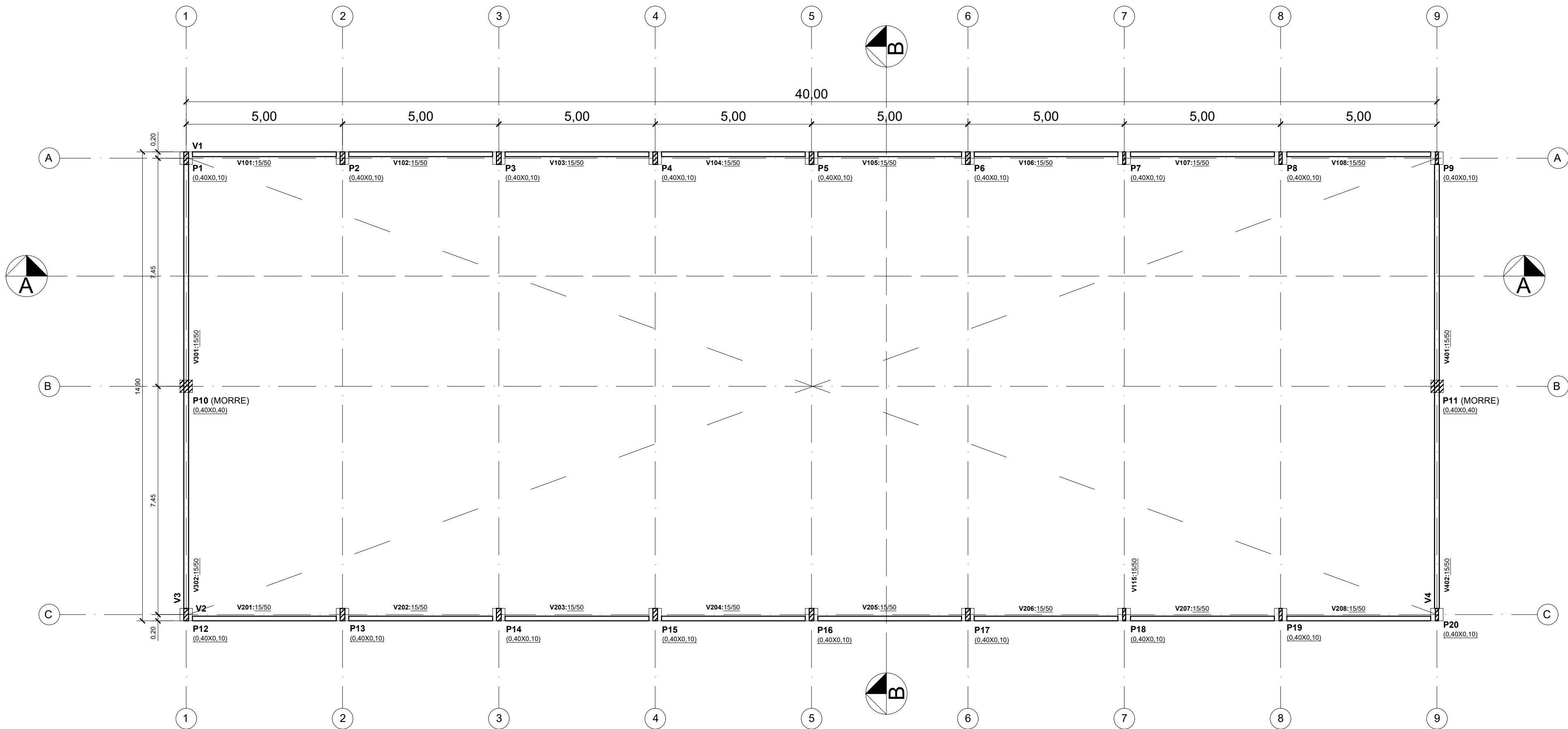
PLANTA FORMA TERREO ESC: 1/100
