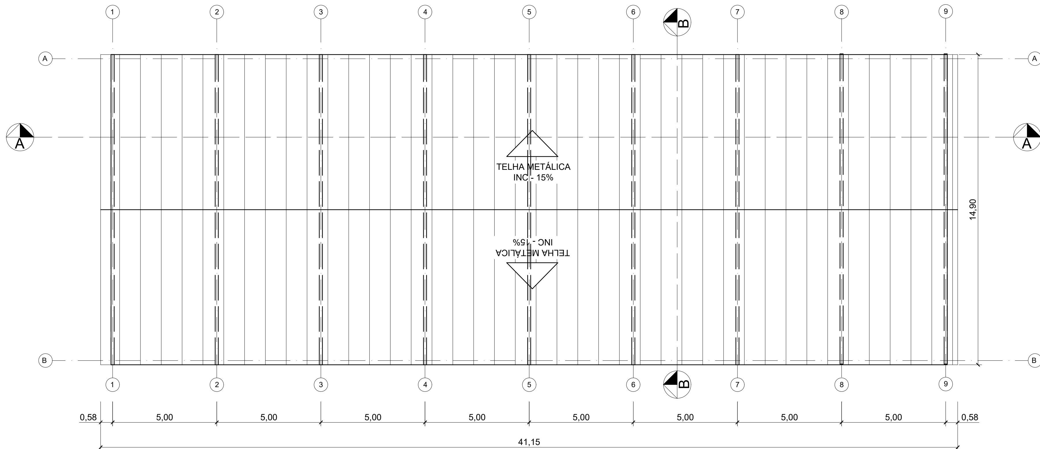
PLANTA DE COBERTURA ESC: 1/100
