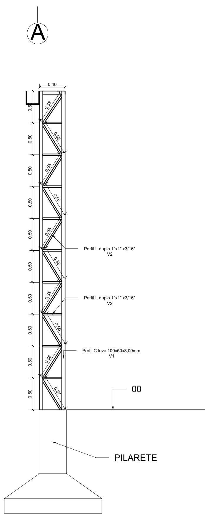
DETALHAMENTO PILAR TRELIÇADO ESC: 1:35
