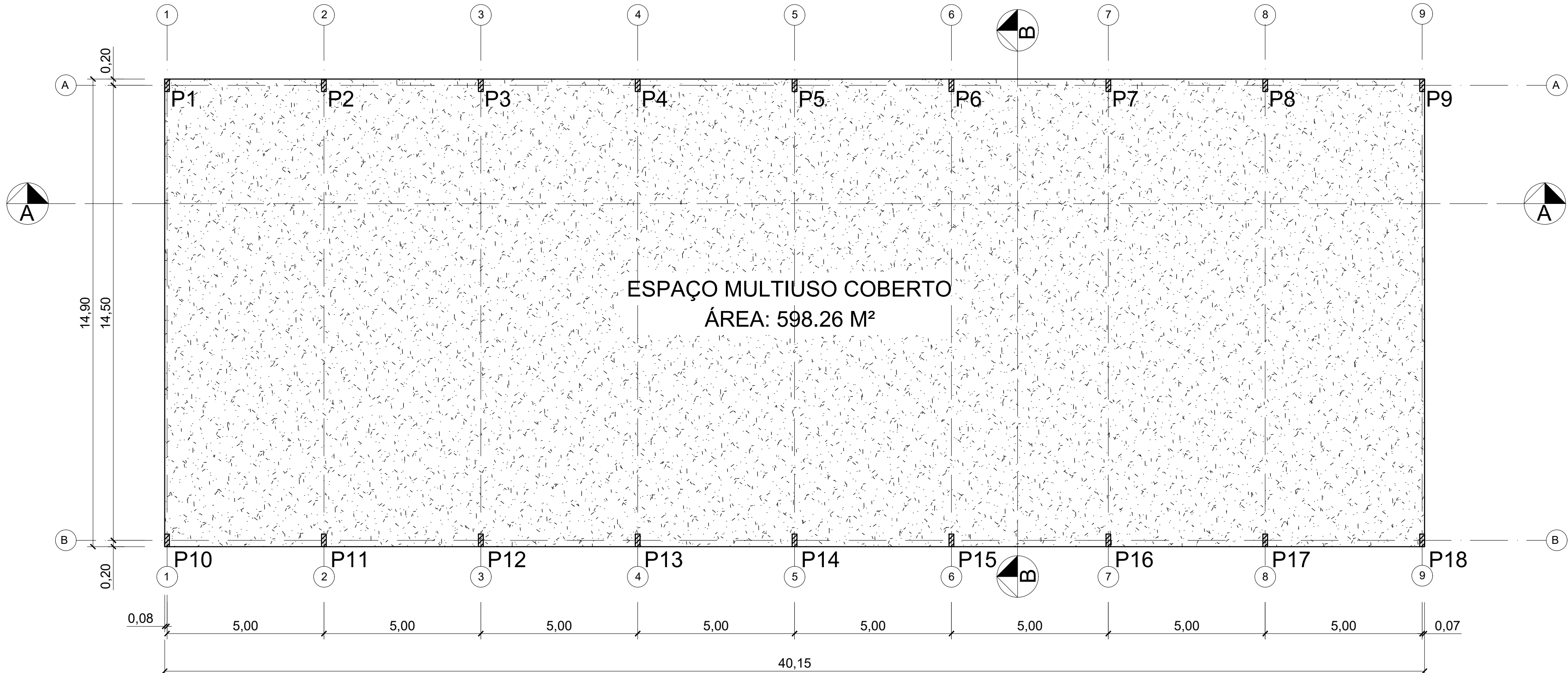
PLANTA BAIXA ESC: 1/100
