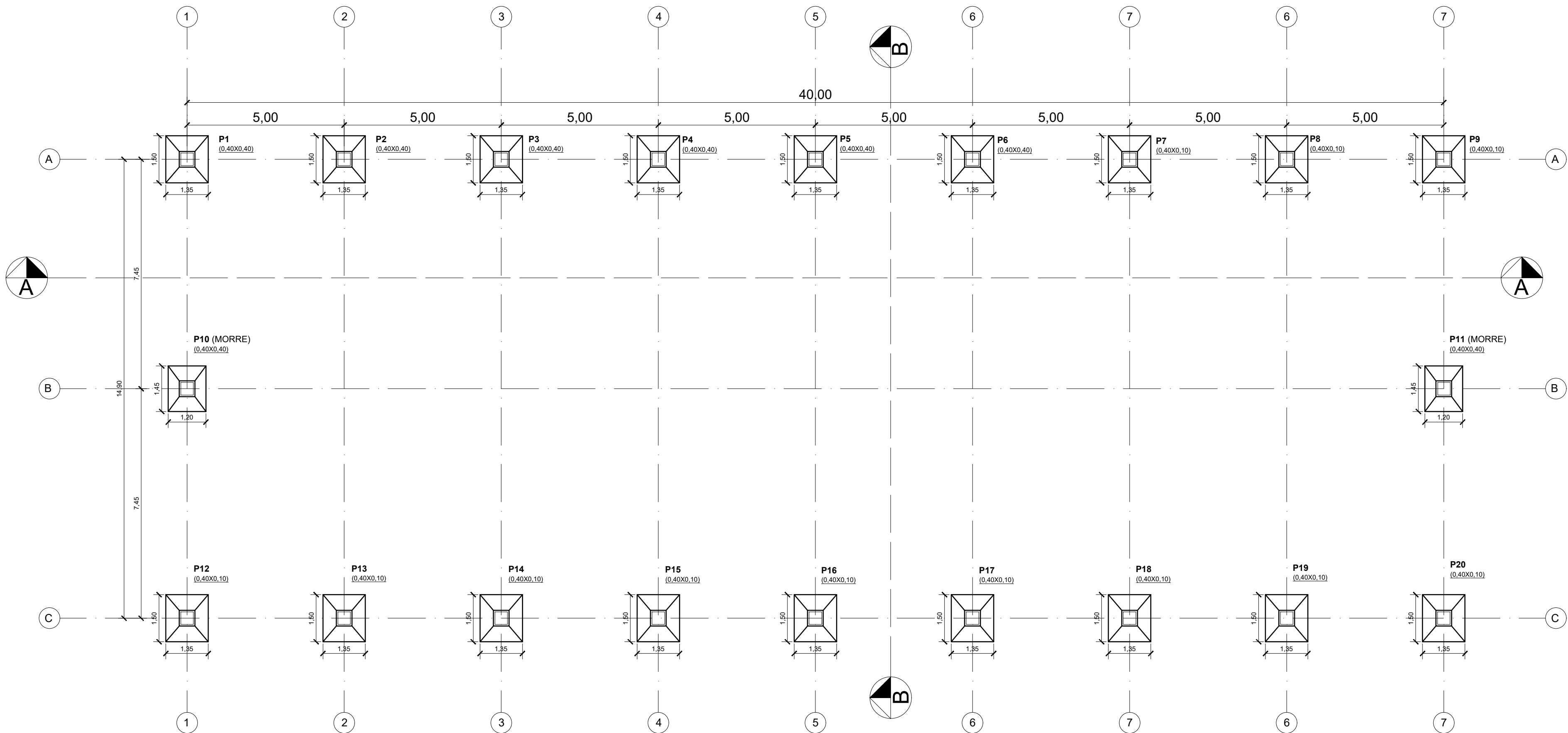
PLANTA FORMA DAS FUNDAÇÕES ESC: 1/100
