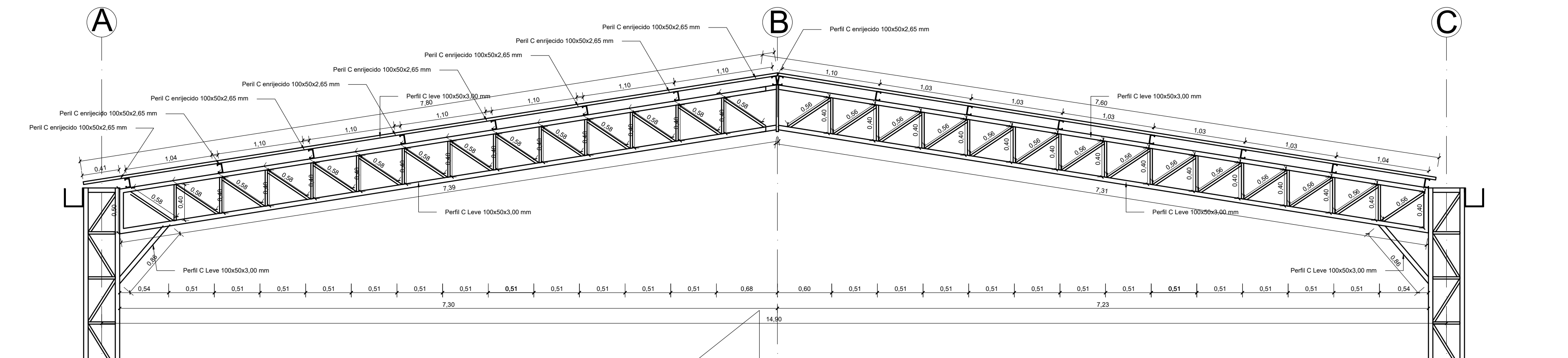
DETALHAMENTO TRELIÇA METÁLICA TIPO ESC: 1:35
