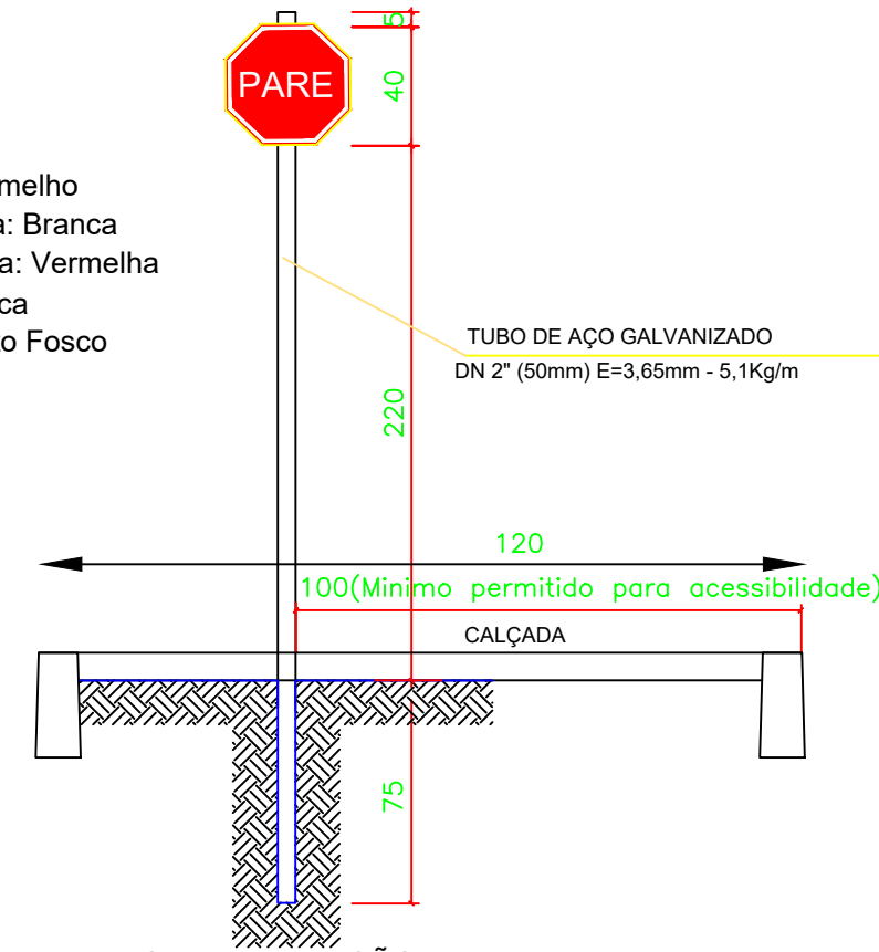
PLACA DE REGULAMENTAÇÃO - 40x40cm PARADA OBRIGATÓRIA - R-1 MEDIDAS EM cm
