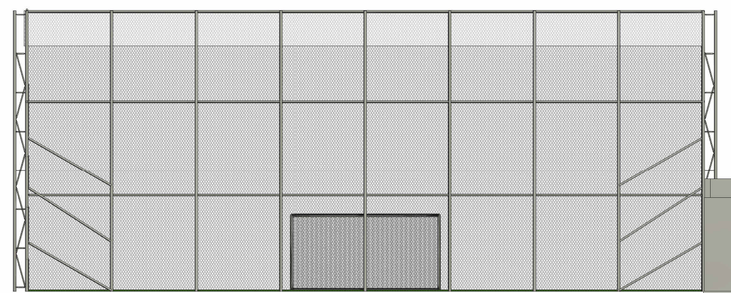
8 FACHADA FUNDOS 1 : 100
