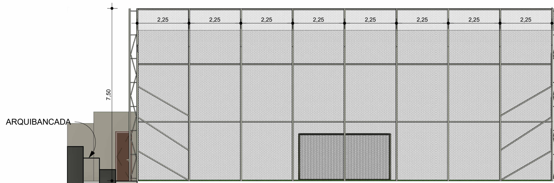
6 CORTE AA 1 : 100
