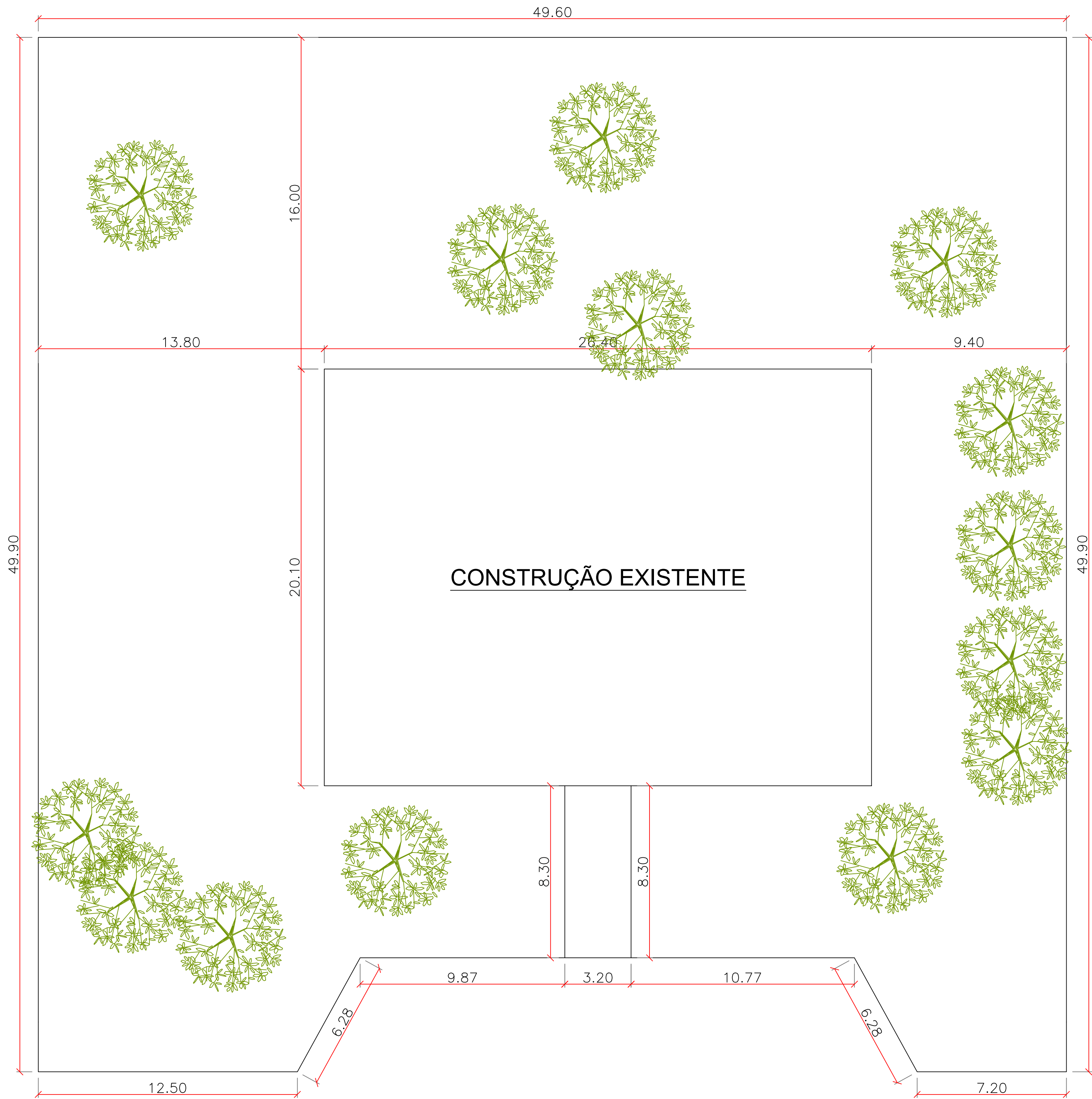
PLANTA BAIXA EXISTENTE esc. 1:100
