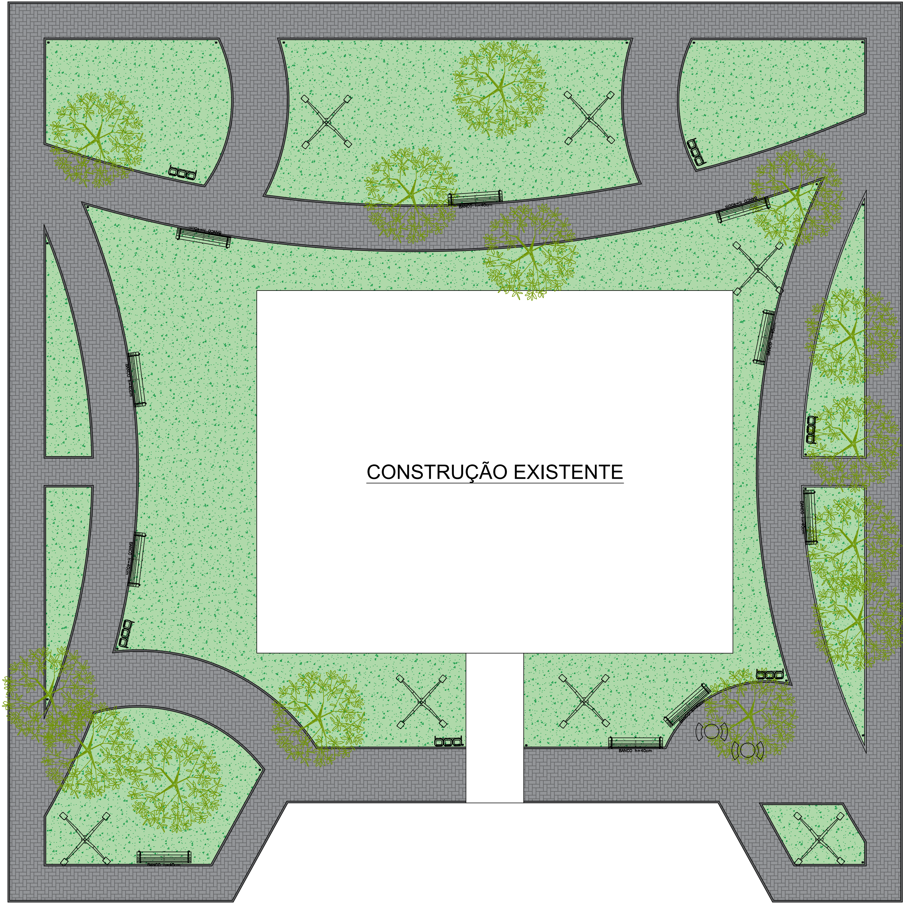
PLANTA BAIXA HUMANIZADA esc: 1:100
