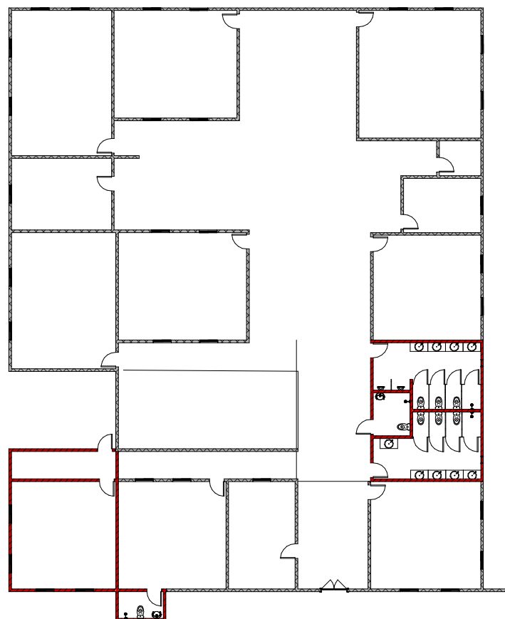
PLANTA BAIXA 2 EXISTENTE/EXECUTAR 1:100
