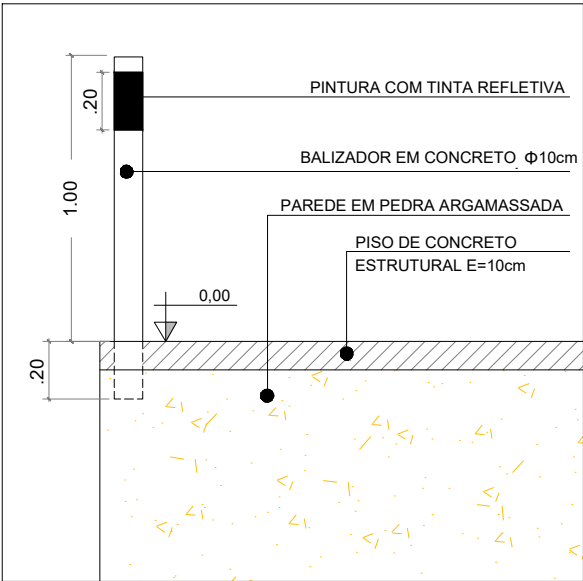
DETALHE DO BALIZADOR ESCALA 1/20
