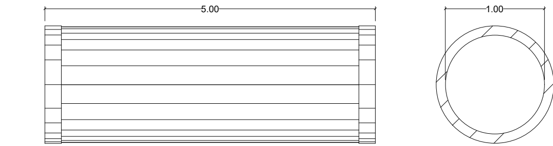
DETALHAMENTO DOS BUEIROS Ø1.00m PLANTA BAIXA E VISTA FRONTAL ESCALA 1/50
