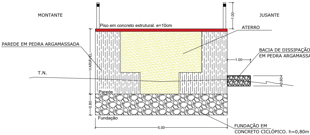
CORTE TRANSVERSAL DA PAREDE ESCALA 1/75
