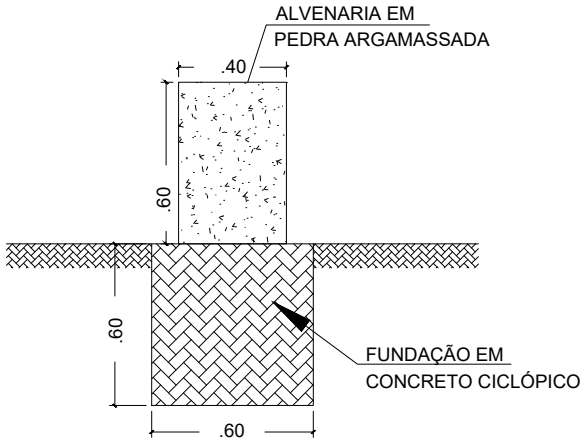
DETALHE DO MURO DE CONTENÇÃO ESCALA 1/20
