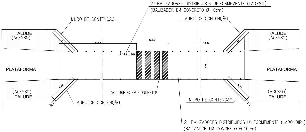
PLANTA BAIXA - PASSAGEM MOLHADA ESCALA 1/125
