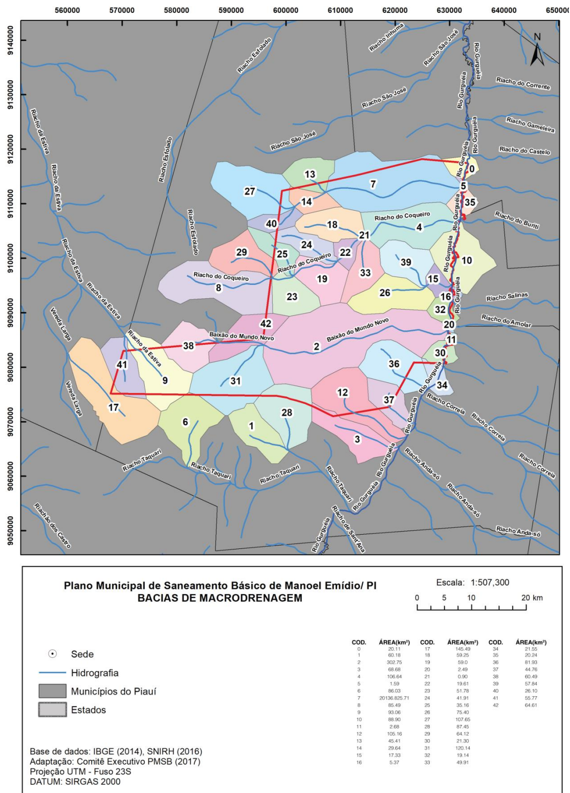
Figura 48 – Bacias de macrodrenagem do município de Manoel Emídio
