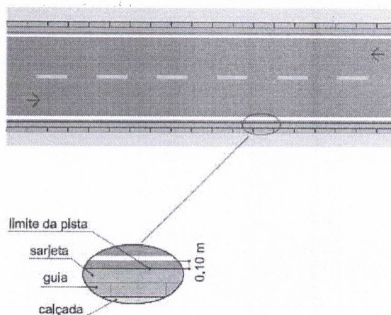
Figura 2. Linha de borda de pista (Manual de Sinalização DNIT, 2010)
