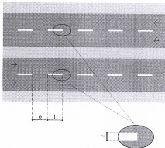
Figura 228 – Linha simples tracejada (LMS-2)
