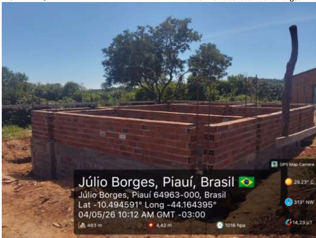
Foto 6: Execução de baldrame
