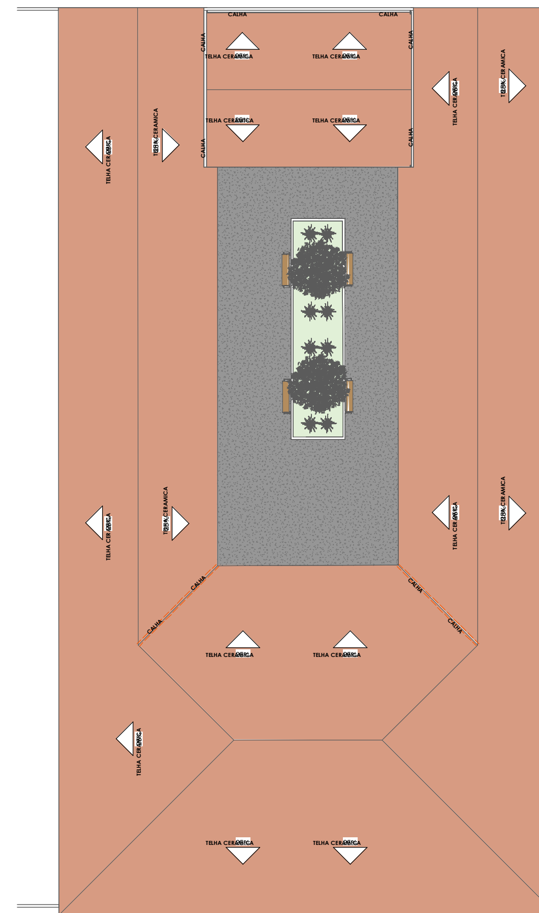
5 COBERTURA E LOCAÇÃO 1:150
