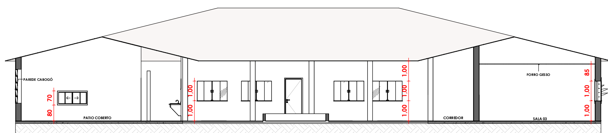
3 Corte 2 1:75
