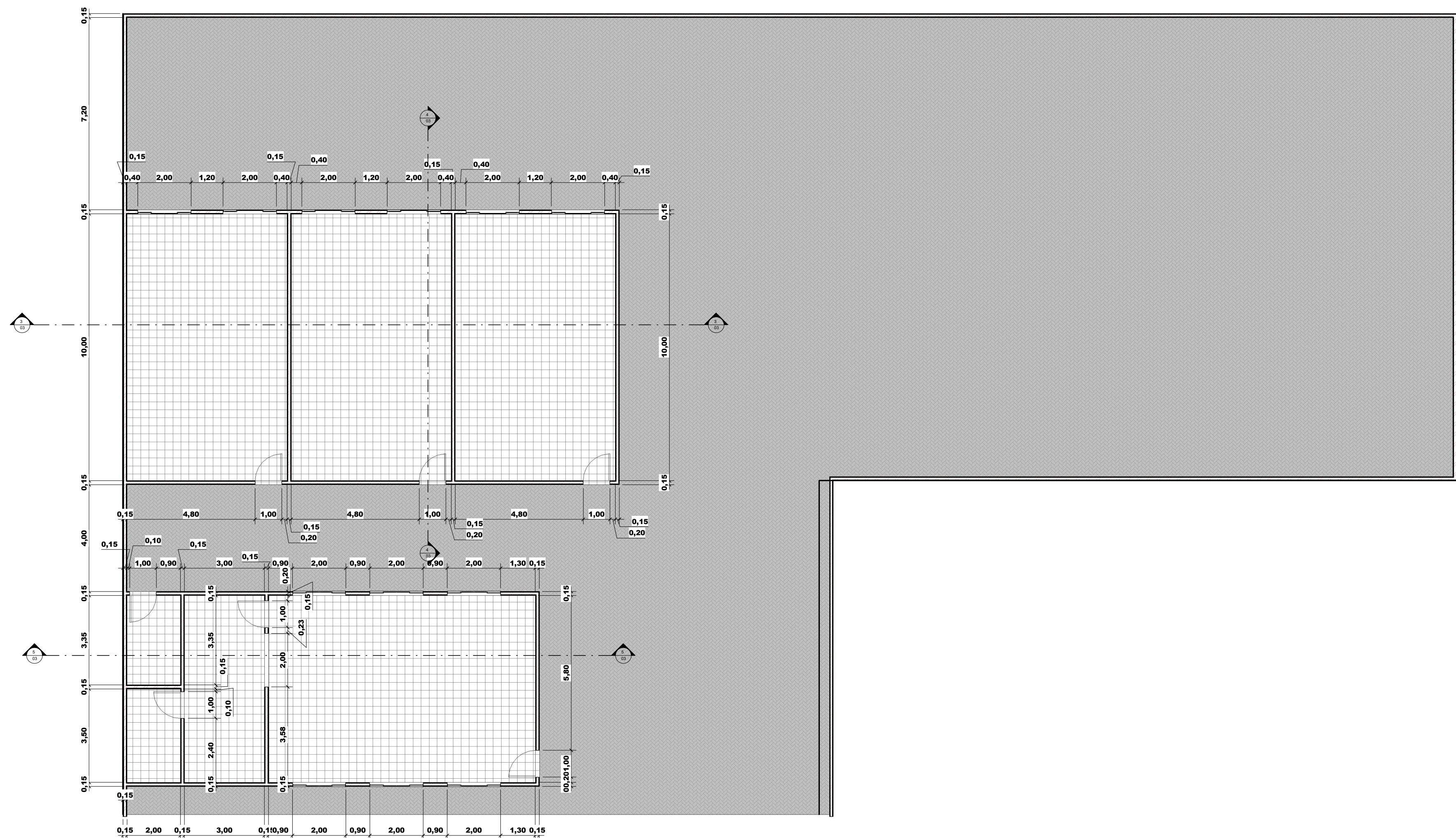
1 PLANTA REFORMA 1 : 75
