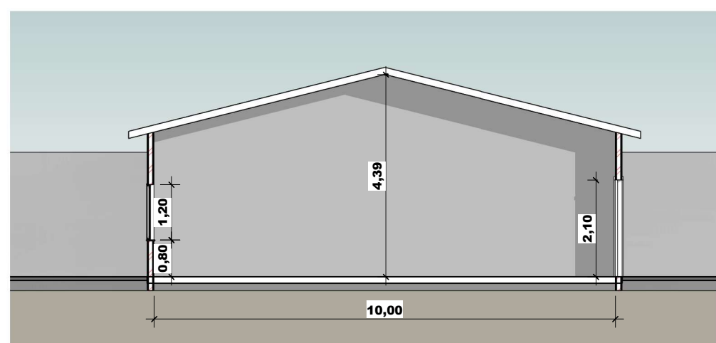
4 CORTE 02 1 : 75
