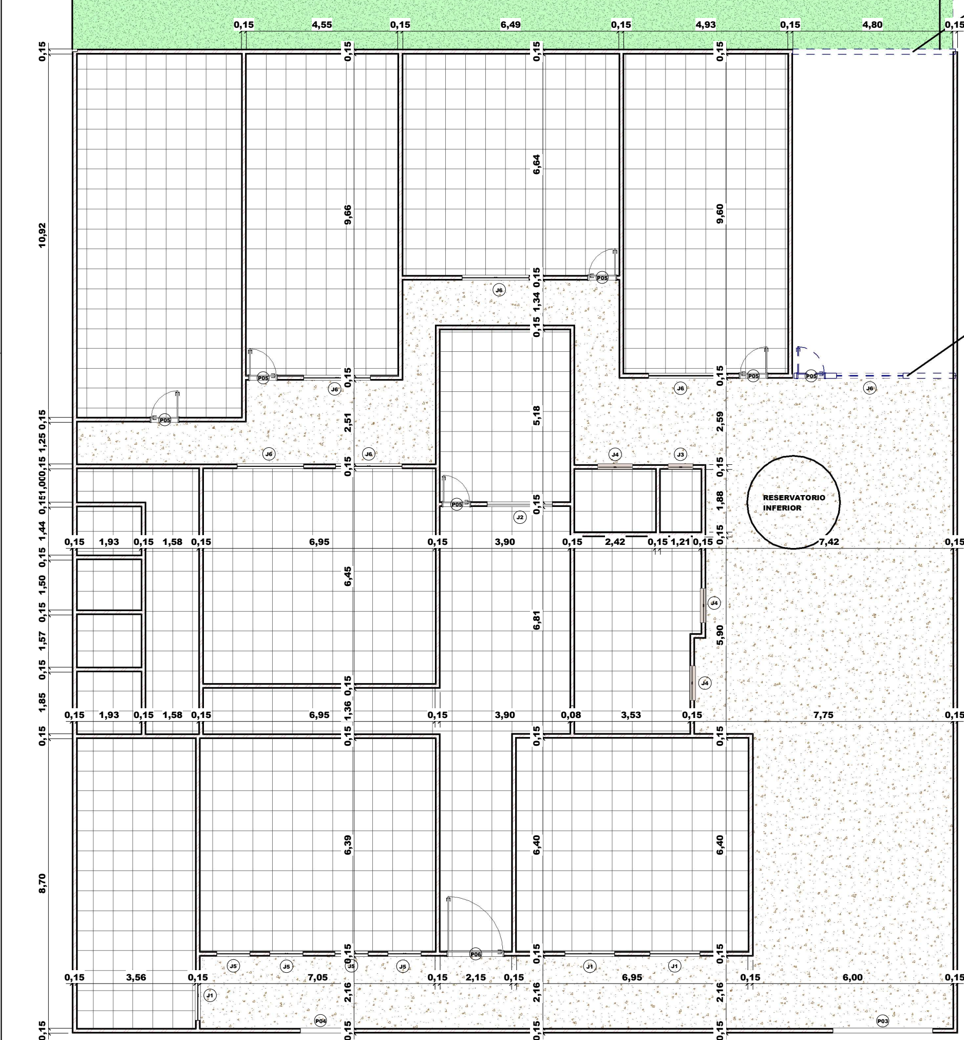
1 PLANTA BAIXA 1 : 75
