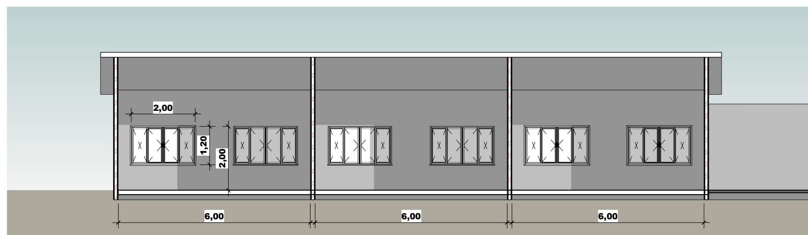
3 CORTE 01 1 : 75
