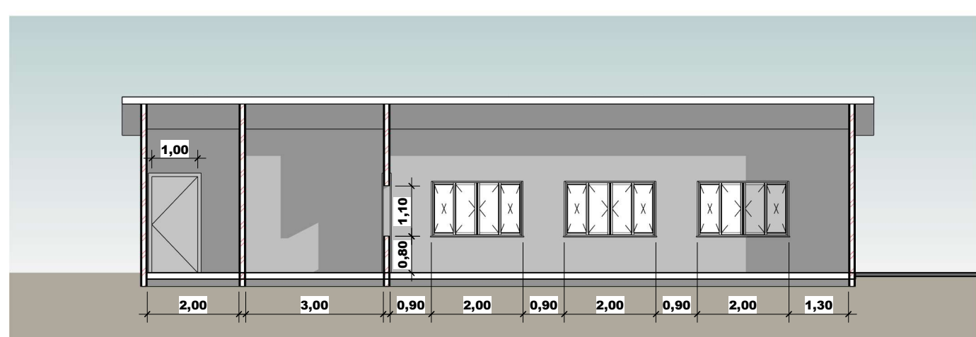
5 CORTE 03 1 : 75
